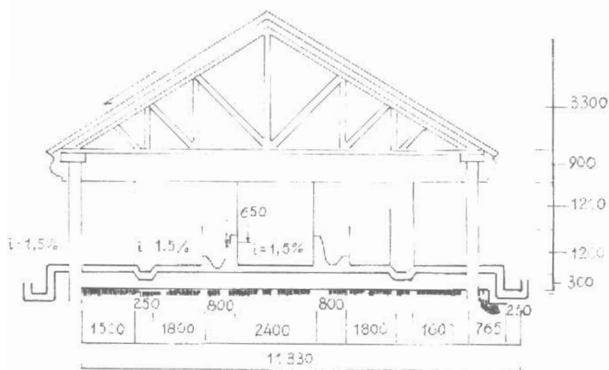
Kiểu chuồng hai dãy đôi đầu có lồi đi giữa (mặt cắt)
