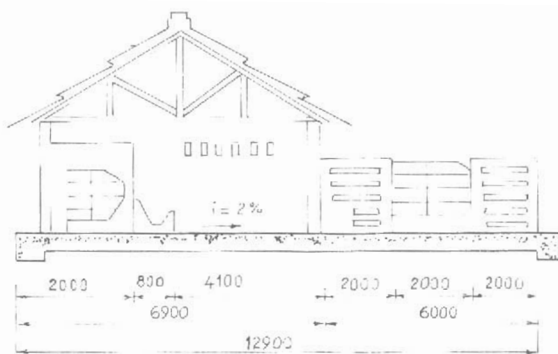
Kiểu chuồng một dãy có lồi đi phía trước máng ăn (mặt cắt)
